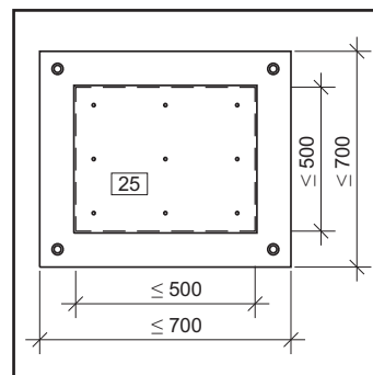
[22] Zugangsklappe
