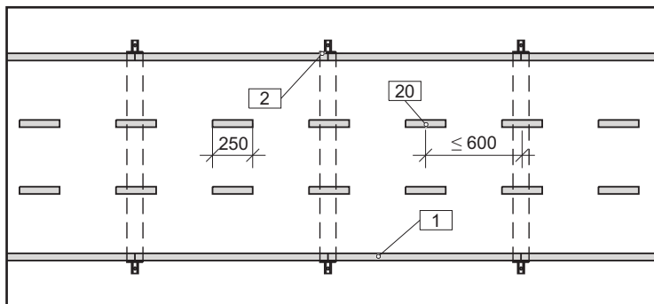
[23] Große Querschnitte mit zwei Aussteifungen
