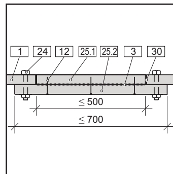
[24] Schnitt Zugangsklappe
