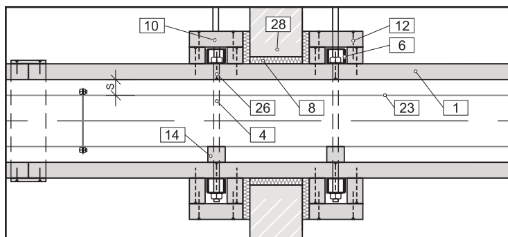
[14] Wanddurchführung
