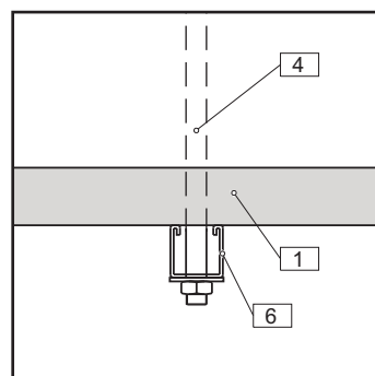
[7] Abhängung, Var. 1
