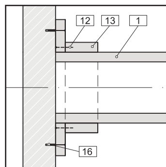
[9] Wandanschluss
